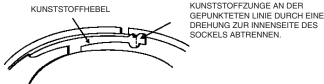
Abbildung 1b: Melderkopf vom Sockel abnehmen
