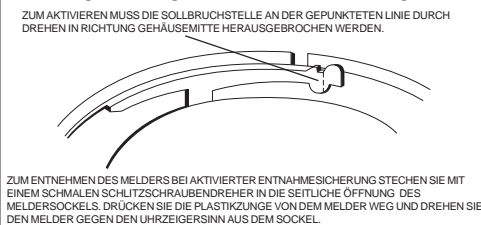
Abbildung 2: Sabotageschutz / Entnahmesicherung
