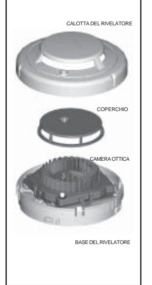
Figura 3: Rivelatore Ottico di Fumo 2351E
