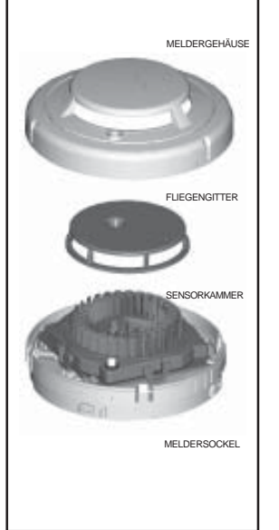
Abbildung 3: 2351E Optischer Rauchmelder
