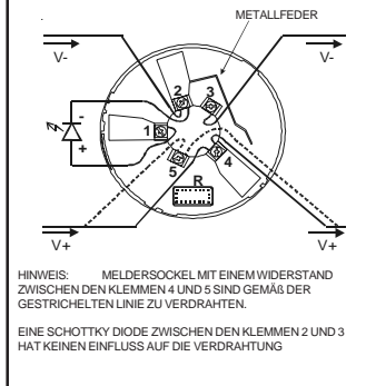
Abbildung 1: Verdrahtung des Meldersockels
