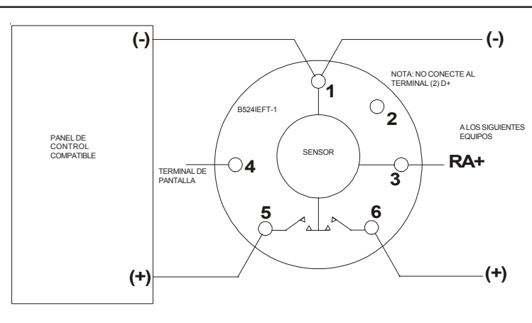
Figura 3. Diagrama de cableado típico
