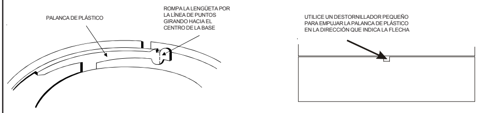
Figura 2. Opción Antimanipulaciones
