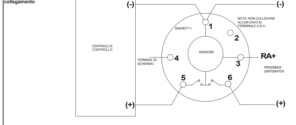
Figura 3. Schema di collegamento
