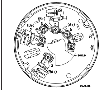
Figura 1. Distribución de los terminales
