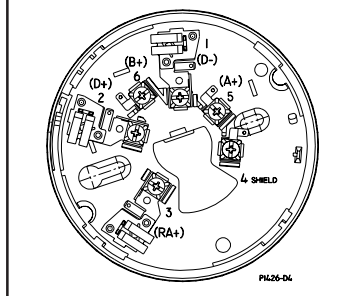
Figura 1. Schema dei terminali
