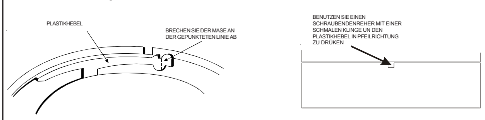
Abb. 2: Diebstahlsicherung
