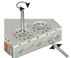
FIGURA 4: CABLAGGIO DEL MODULO A USCITA SINGOLA E DOPPIO INGRESSO M221E
