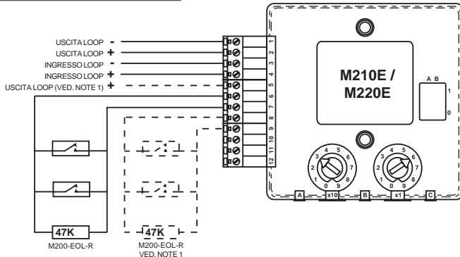
FIGURA 3: CABLAGGIO DEL MODULO A INGRESSO SINGOLO M210E E A INGRESSO DOPPIO M220E
