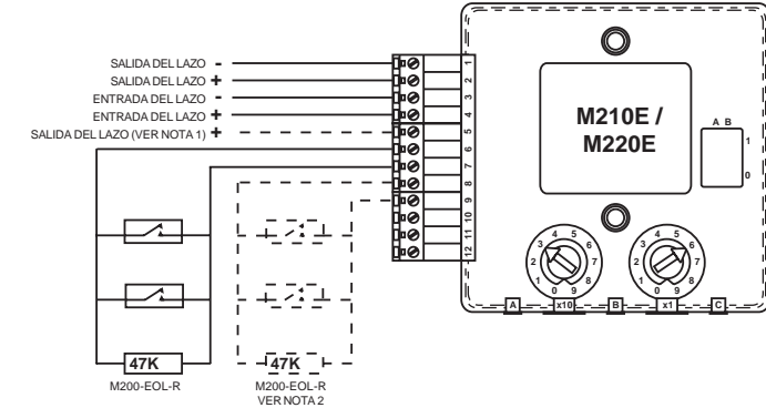
FIGURA 3: CONEXIONES DE LOS MÓDULOS M210E DE ENTRADA ÚNICA Y M220E DE ENTRADA DOBLE
